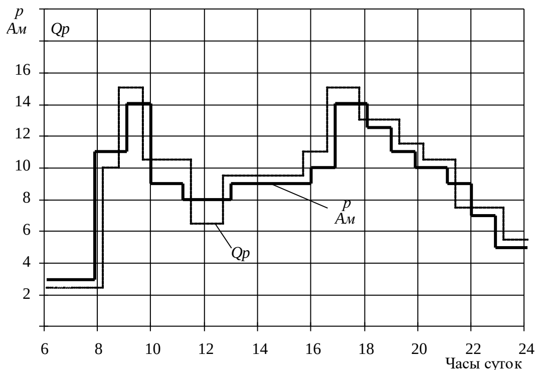
Рис. 7. Расчётная диаграмма потребности в автобусах
