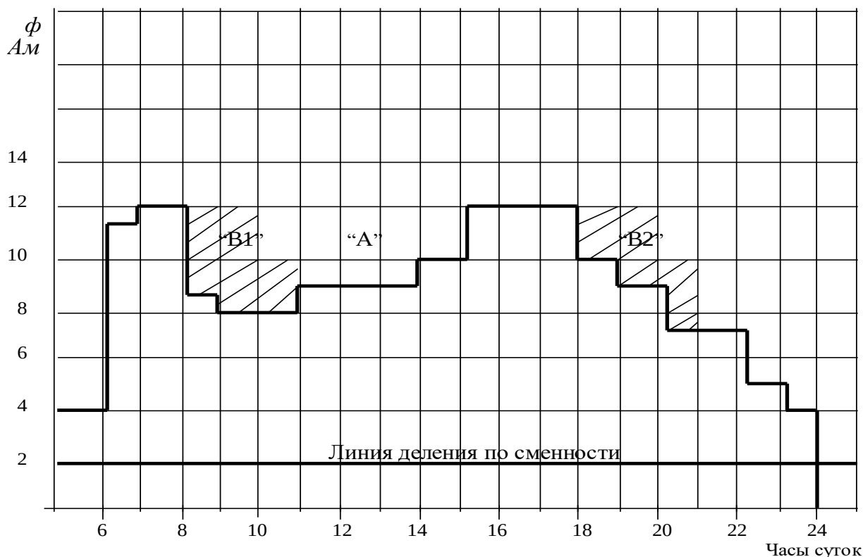
Рис. 9. Диаграмма набора обеденных перерывов
