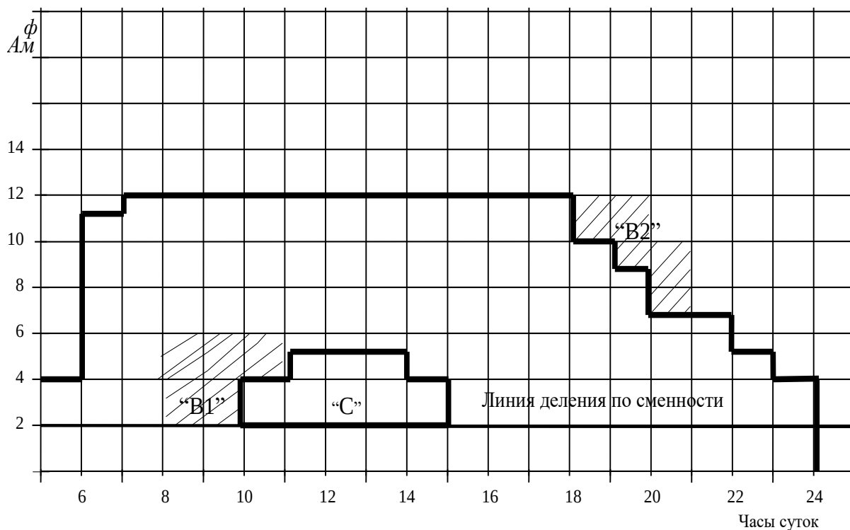
Рис. 10. Диаграмма распределения автобусов по сменности и режиму работы
