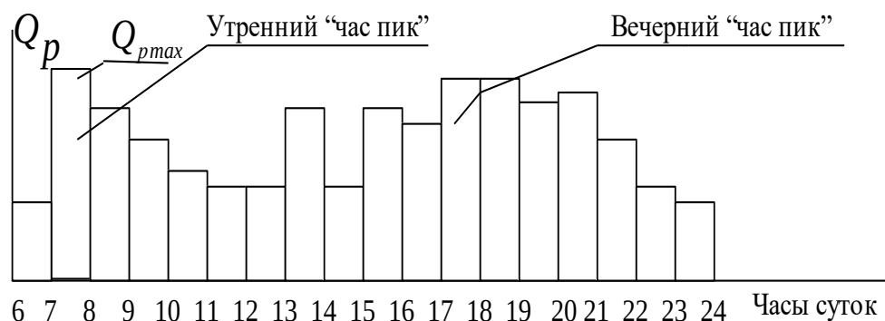
Рис. 3. Эпюра расчетных величин пассажиропотока по часам суток
