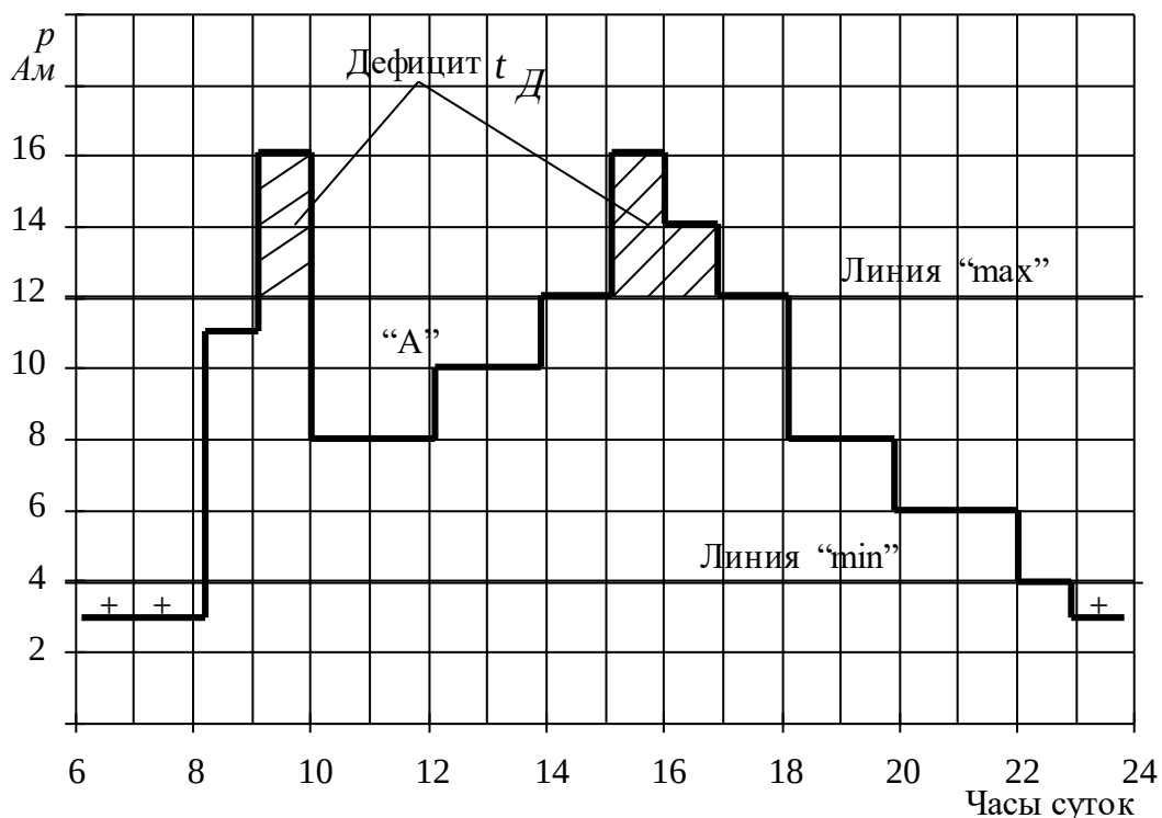
Рис. 8. Диаграмма «максимум» потребности в автобусах
